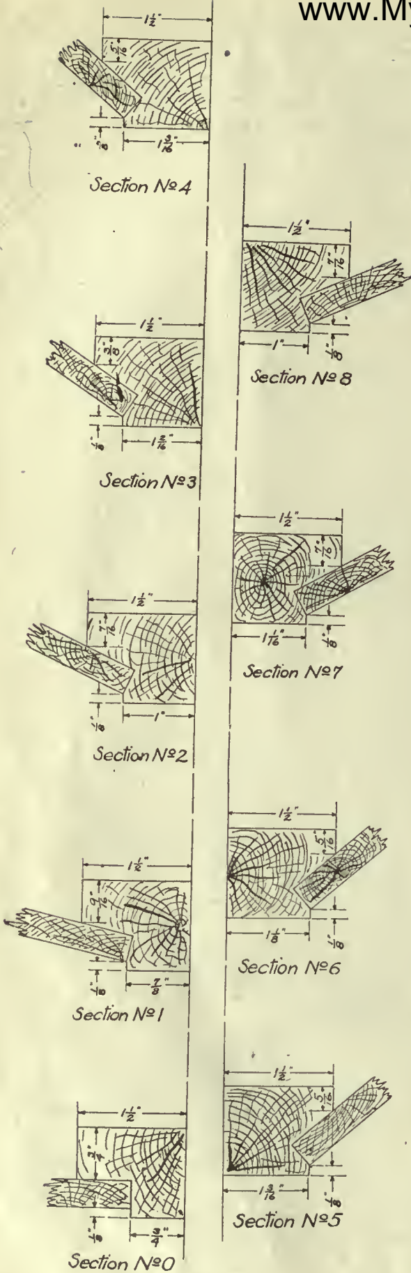
KEEL SECTIONS
