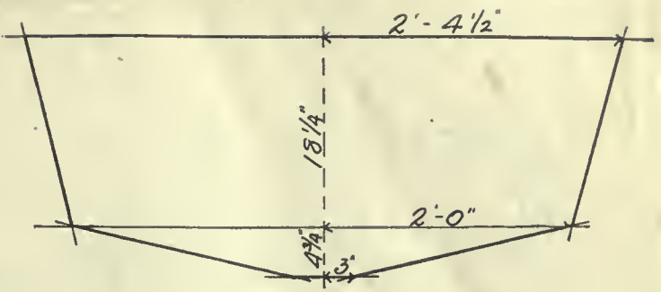
Mould No-2.
