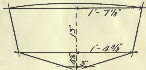
Transom.
