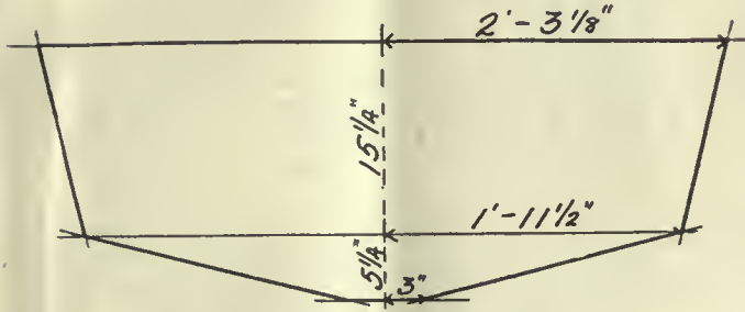
Mould No-3
