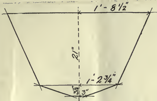
Mould No-1.
